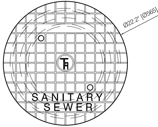
LID
